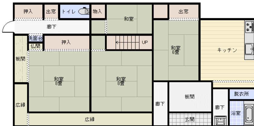
(間取り図) 1階
