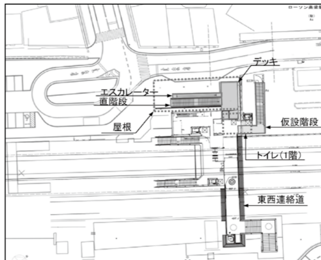
付け替えが計画されている東西連絡道の西側階段の形状
