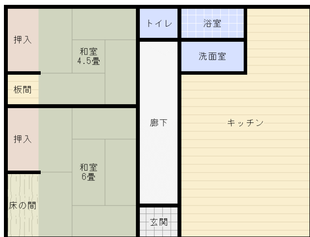
(間取り図)
