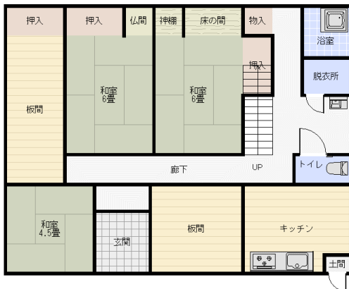
間取り図 (1階)
