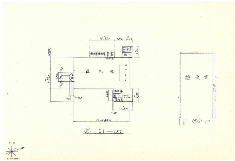
平面図②
