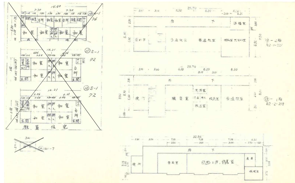
平面図①
