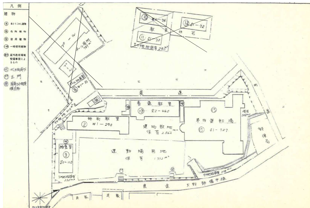
配置図
