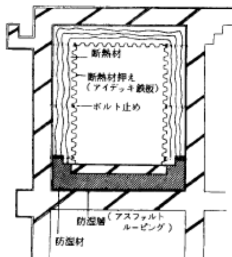
図6—2 冷凍室等断熱処理施工例
