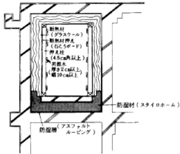
図6—1 冷凍室等断熱処理施工例
