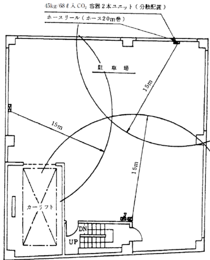
平面図
