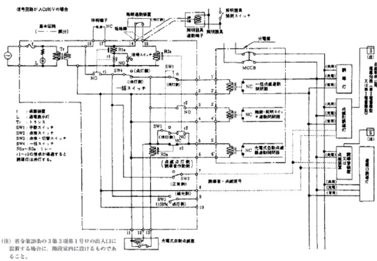
図16-22 機器結線図
