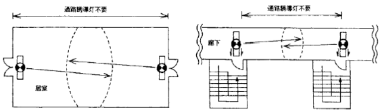
図16-19 通路誘導灯の設置不要例
