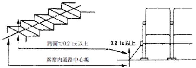
図16-21 客席誘導灯の設置例
