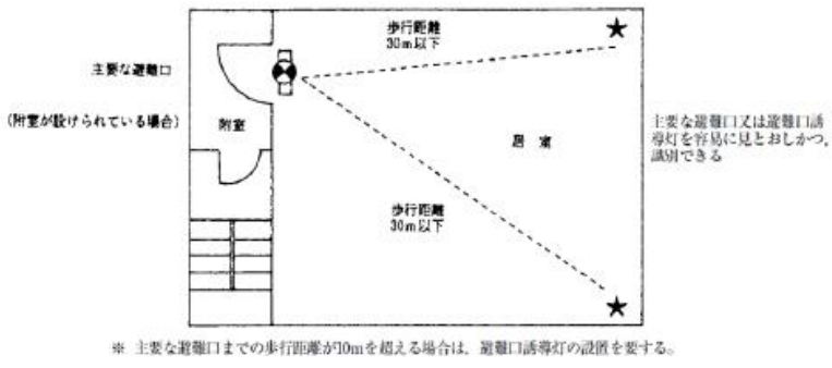
図16-6 通路誘導灯の設置を要しない場合
